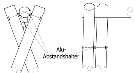
Anordnung Alu-Abstandshalter
